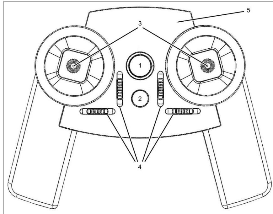
Abb. 1: Oberseite des Senders
