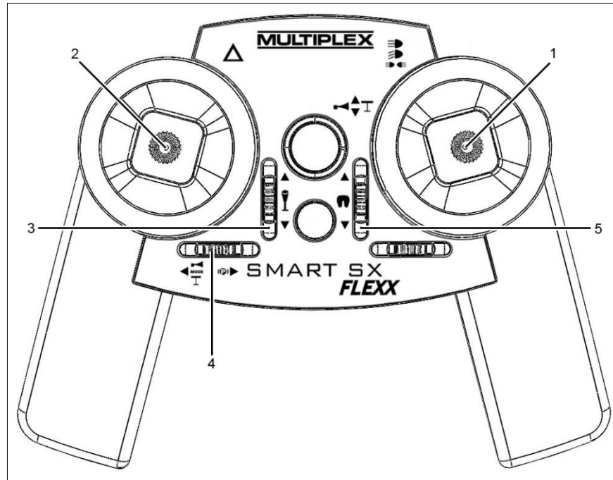
Fig. 4: Trasmettitore SMART SX FLEXX – Assegnazione per modelli di autocarri
