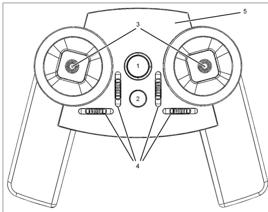
Fig. 1 : Face supérieure de l'émetteur
