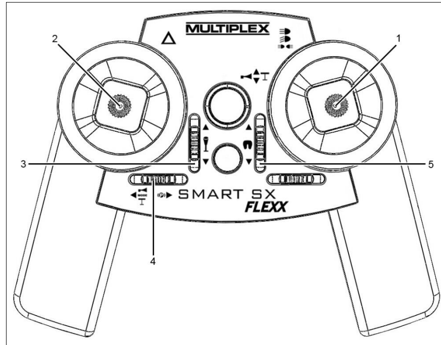
Fig. 4: emisora SMART SX FLEXX: asignación para modelos de camiones
