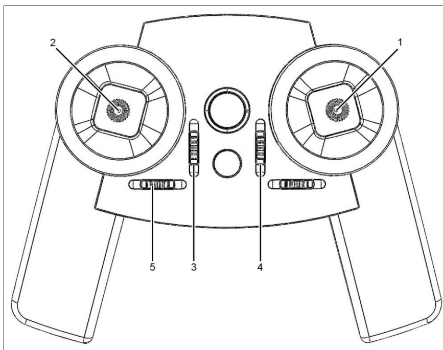
Fig. 6: Trasmettitore SMART SX FLEXX – Interruttori e attribuzione dei servi
