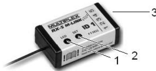
Abb. 3: Empfänger RX-5 light M-LINK ID 1
