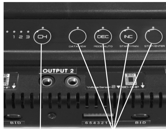
„CH“- Taste
